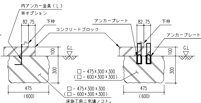
C ~ C' 断面 (内アンカー用)
