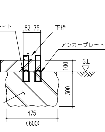
D ~ D' 断面 (外アンカー用)
