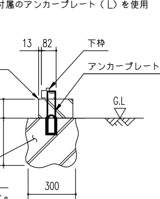
B ~ B' 断面 (外アンカー用)
