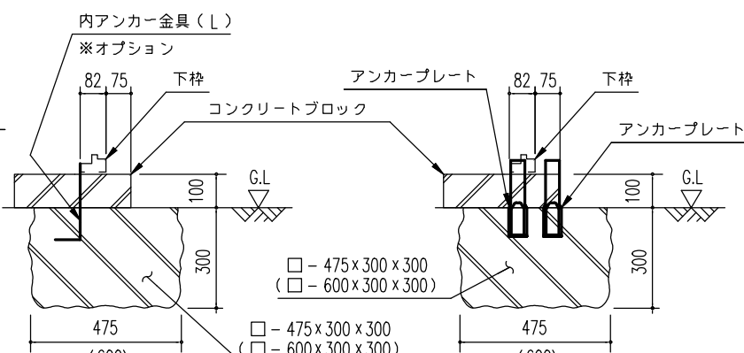
B ~ B' 断面 (外アンカー用)
