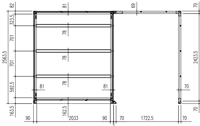
床 伏 図 (S = 1/50)
