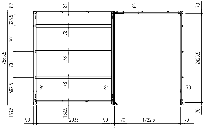
床伏図 (S = 1/50)
