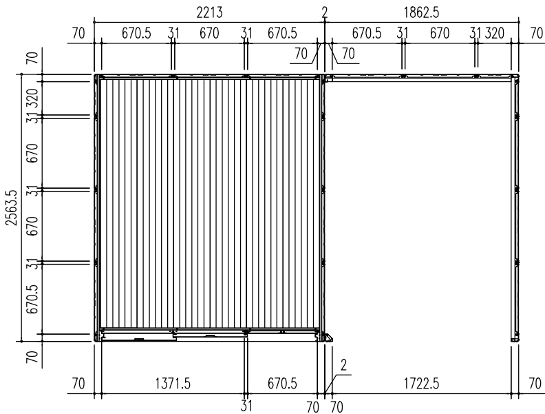
平面図 (S = 1/50)
