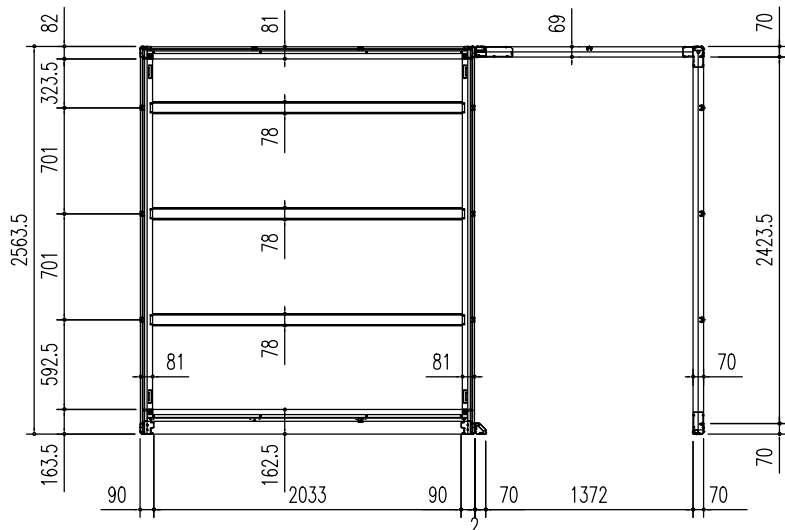
床伏図 (S = 1/50)
