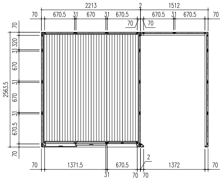
平面図 (S = 1/50)
