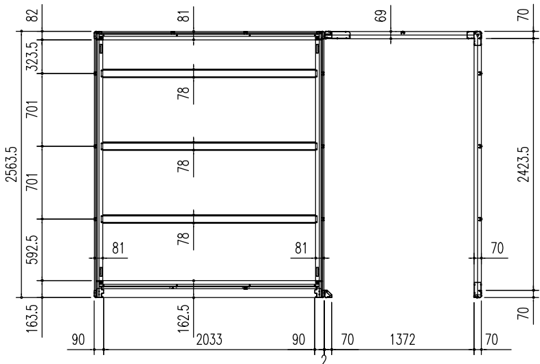
床伏図 (S = 1/50)
