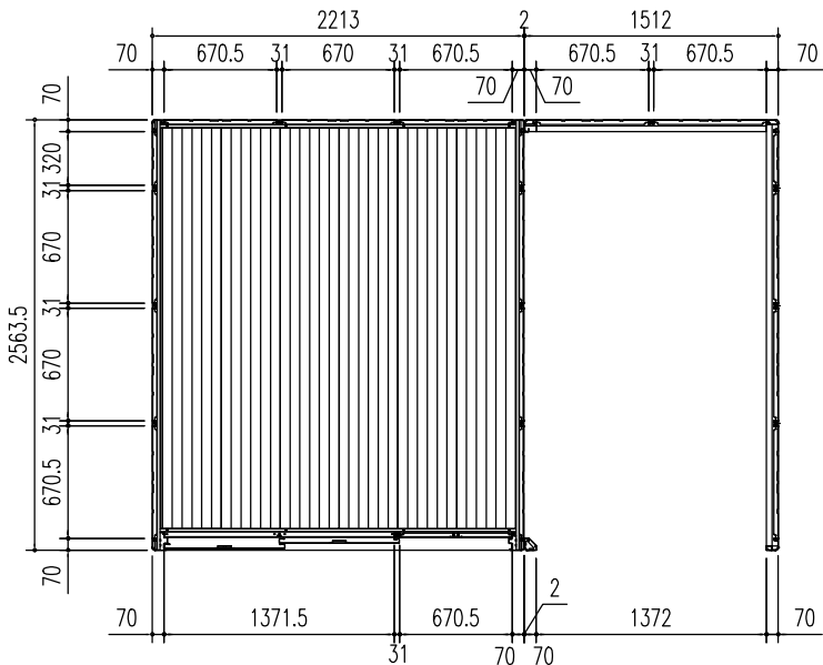
平面図 (S = 1/50)
