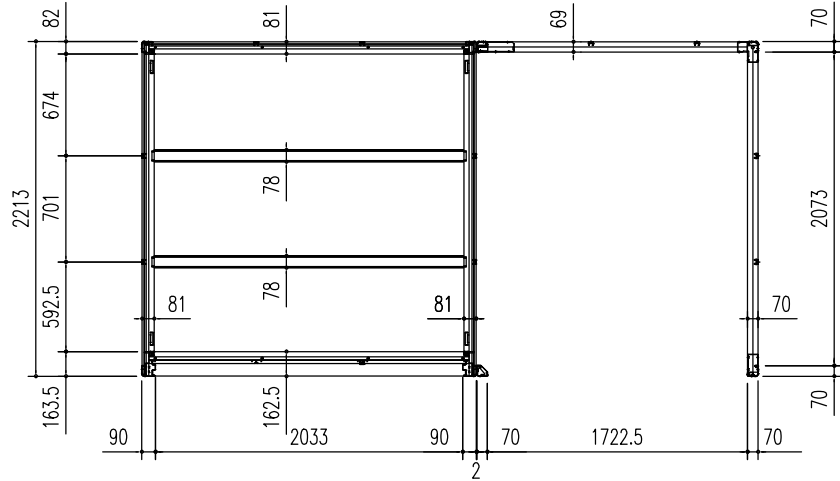
床 伏 図 (S=1/50)
