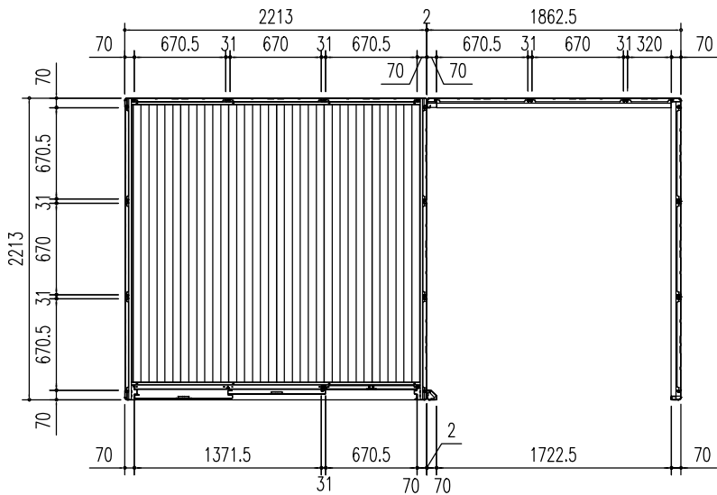
平 面 図 (S = 1/50)
