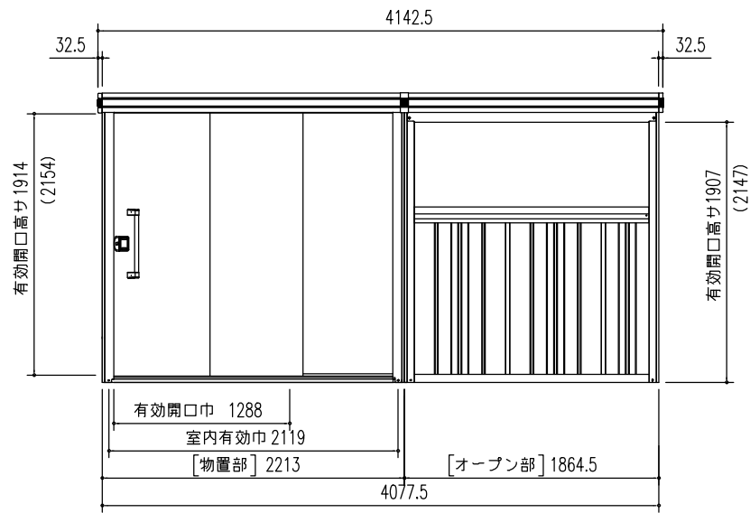
正面立面図 (S = 1/50) ※ ( ) 内寸法は、Hタイプを示す。
