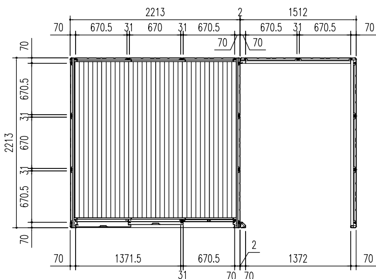
平面図 (S = 1/50)
