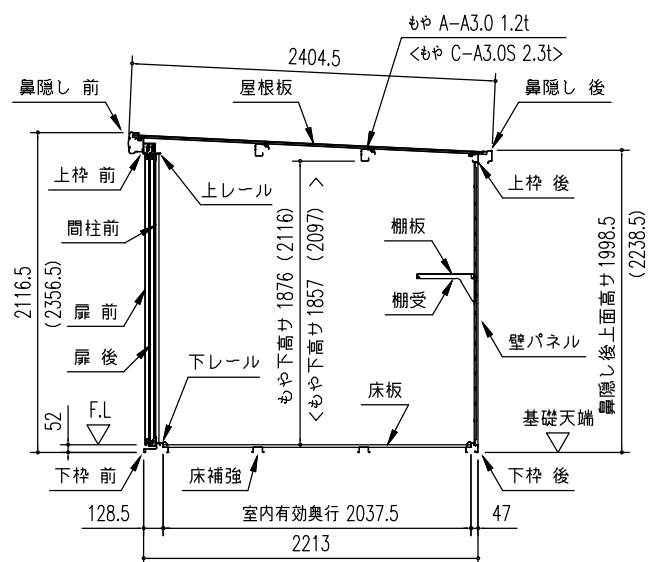
「物置部」矩計図 (S = 1/50) ※ ( ) 内寸法は、Hタイプを示す。 ※ <>内は横雪型を示す。
