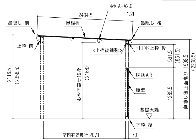
「オープン部」矩計図 (S = 1/50) ※ ( ) 内寸法は、Hタイプを示す。 ※ <>内は横雪型を示す。
