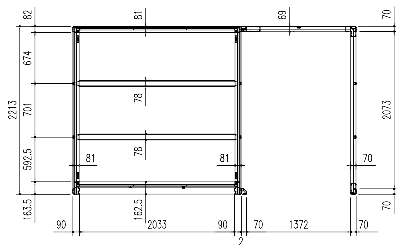
床伏図 (S = 1/50)
