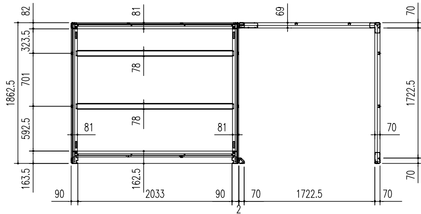
床伏図 (S = 1/50)
