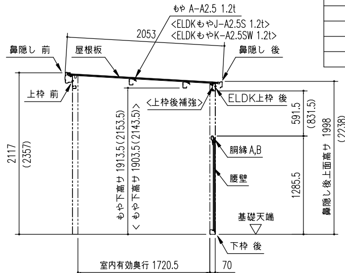
※ ( ) 内寸法は、Hタイプを示す。 ※ <>内は積雪型を示す。
