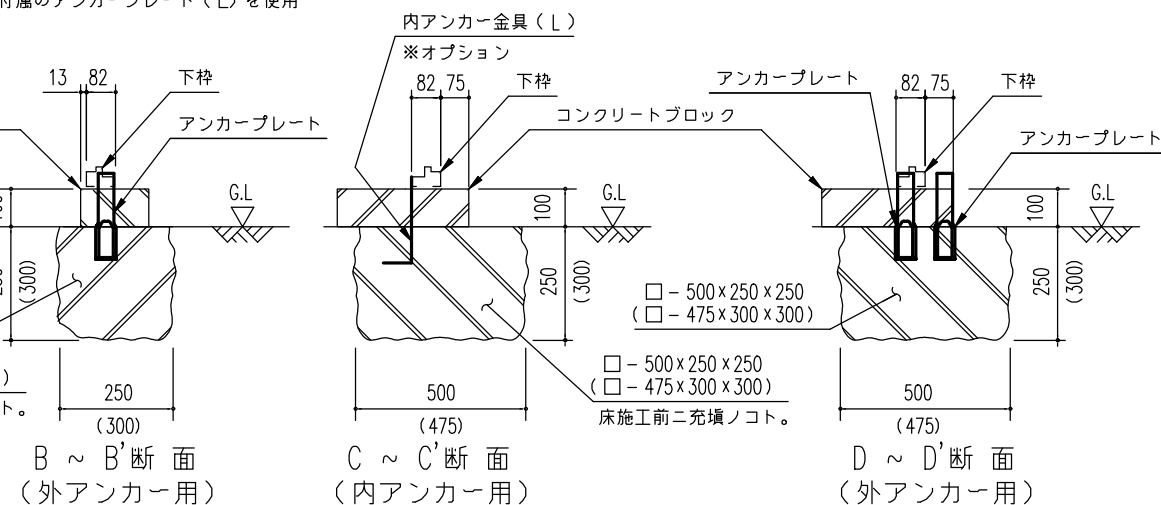
ブロック基礎断面図例 (S=1/20)
