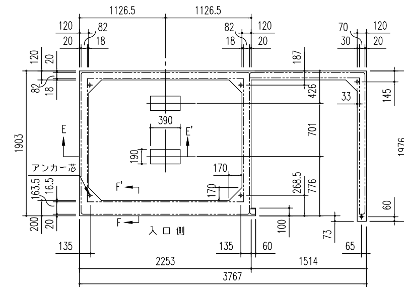
布基礎伏図 (S=1/50)
