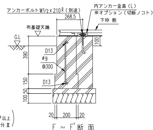
F ~ F' 断面
