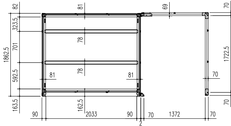
床伏図 (S=1/50)
