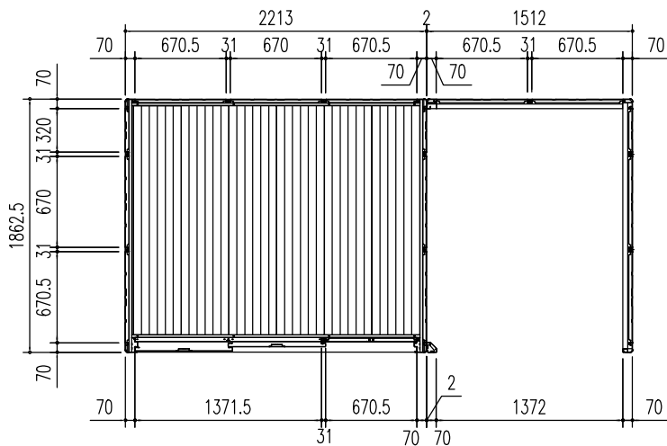
平面図 (S=1/50)
