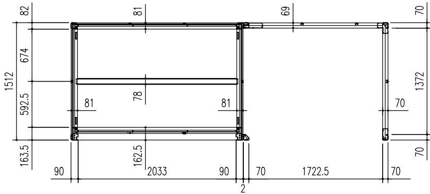
床 伏 図 (S= 1/50)
