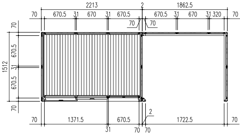
平 面 図 (S= 1/50)
