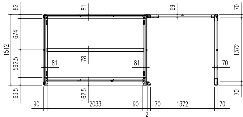
床伏図 (S=1/50)
