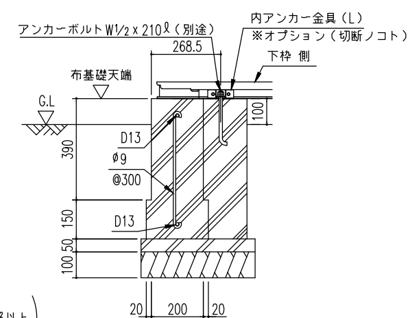
布基礎断面図例 (S=1/20)
