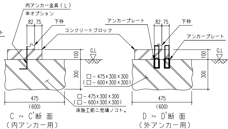
ブロック基礎断面図例 (S=1/20)
