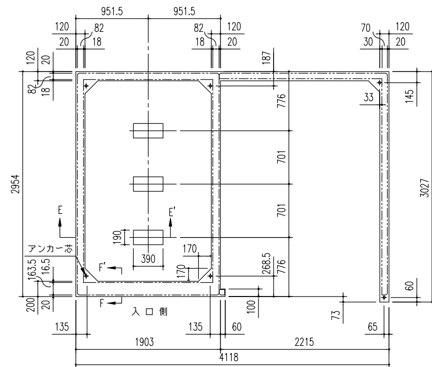
布基礎伏図 (S=1/50)
