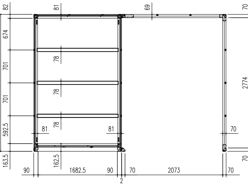
床伏図 (S=1/50)
