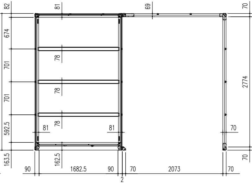
床伏図 (S=1/50)
