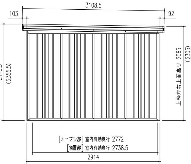
側面立面図 (S=1/50) ※( ) 内寸法は、Hタイプを示す。
