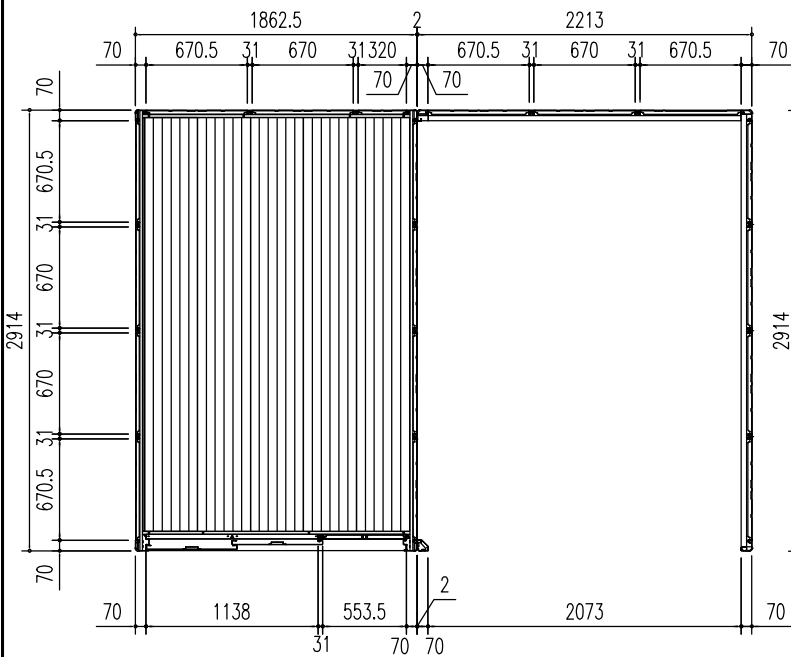
平面図 (S=1/50)
