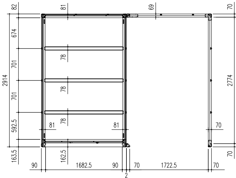
床伏図 (s = 1/50)
