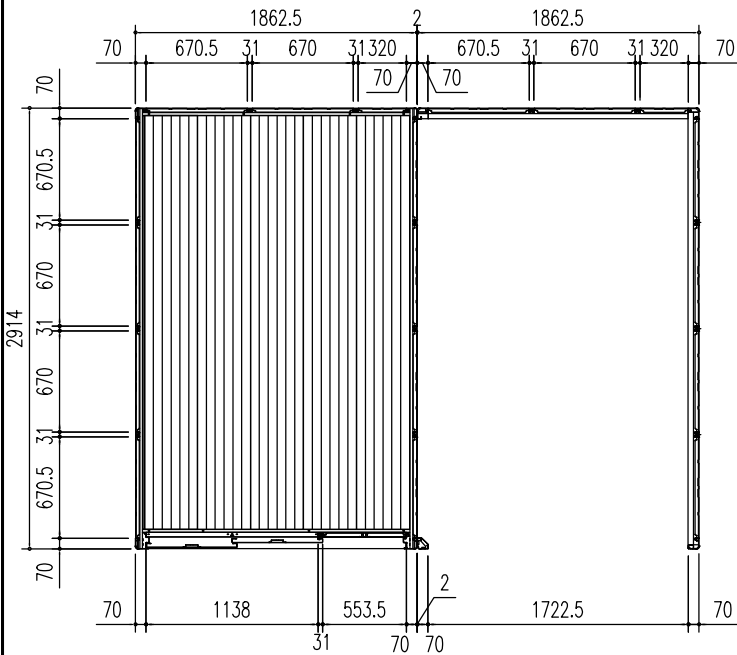
平面図 (S=1/50)
