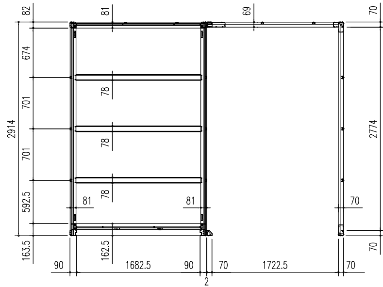
床伏図 (S=1/50)
