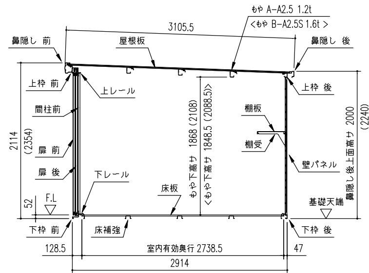
〔物置部〕矩計図 (S=1/50) ※ ( ) 内寸法は、Hタイプを示す。 ※ <>内は積雪型を示す。
