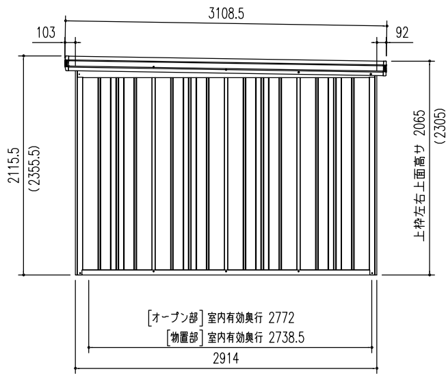
側面立面図 (S=1/50) ※ ( ) 内寸法は、Hタイプを示す。
