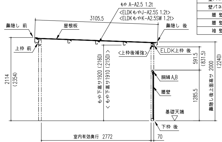
〔オープン部〕矩計図 (S=1/50) ※ ( ) 内寸法は、Hタイプを示す。 ※ <>内は積雪型を示す。
