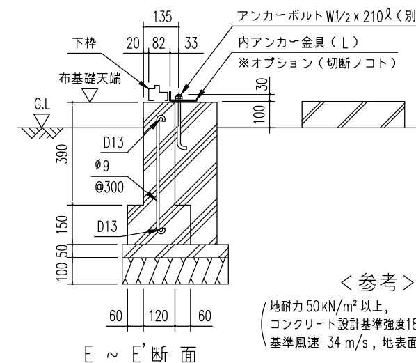
布基礎断面図例 (S=1/20)
