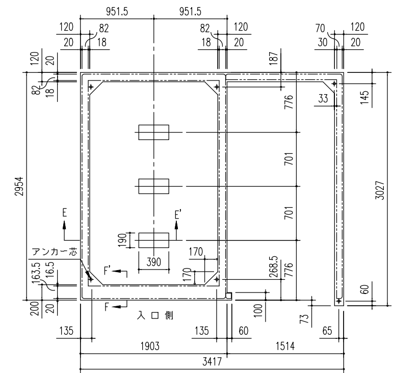
布基礎伏図 (S=1/50)
