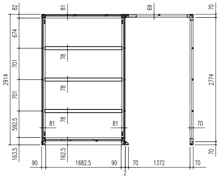
床伏図 (S = 1/50)
