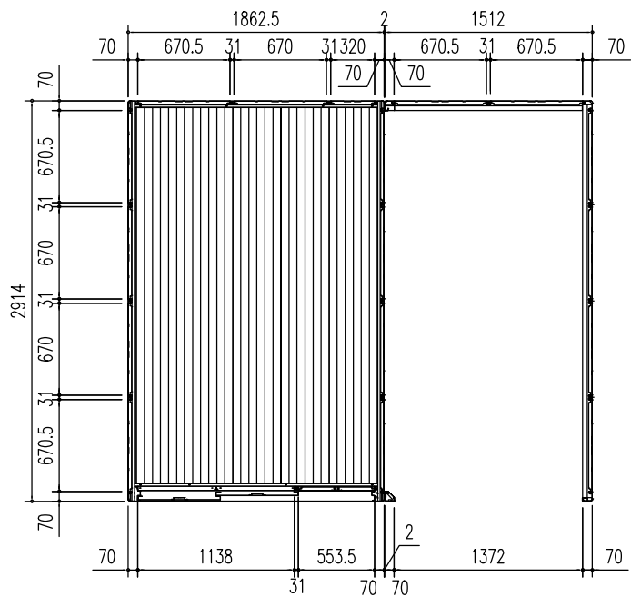
平面図 (S = 1/50)
