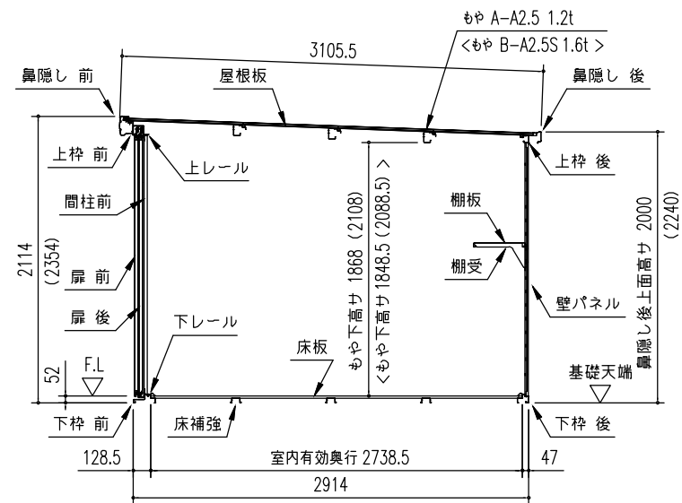
〔物置部〕矩計図 (S = 1/50)
