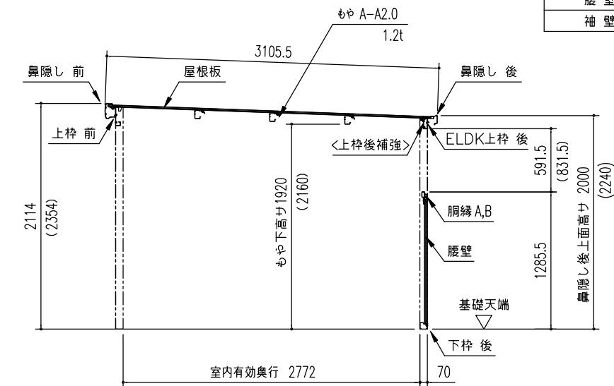
〔オープン部〕矩計図 (S = 1/50)
