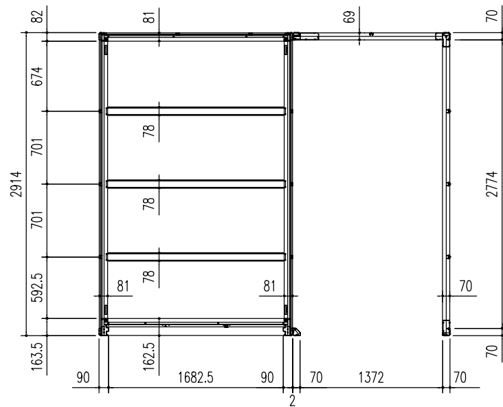
床伏図 (S = 1/50)
