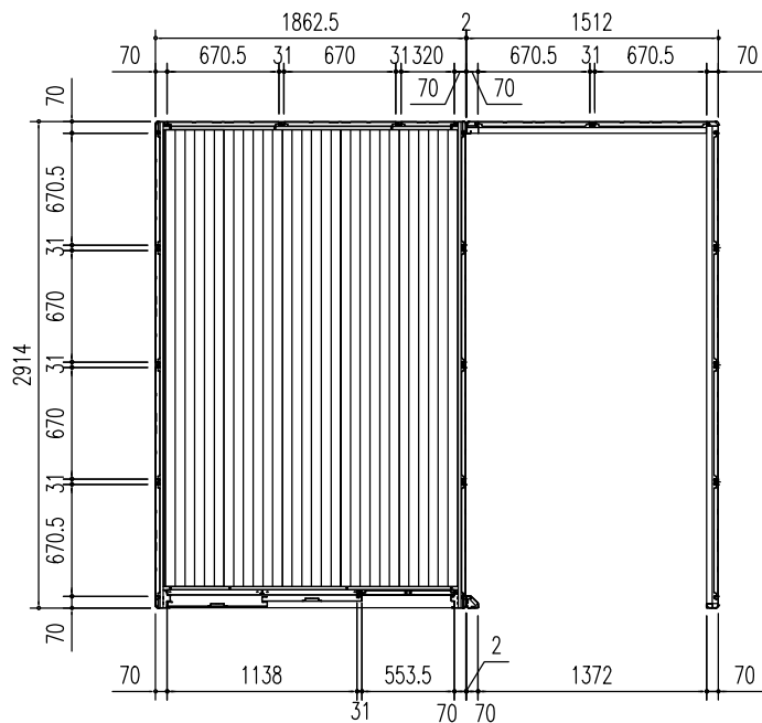
平面図 (S = 1/50)
