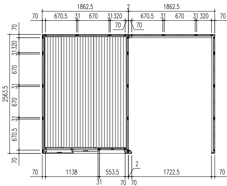
平面図 (S=1/50)
