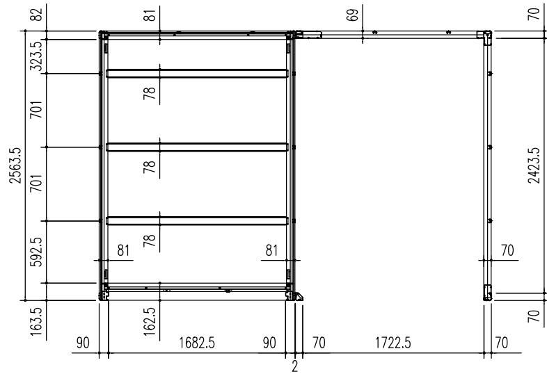
床伏図 (S=1/50)
