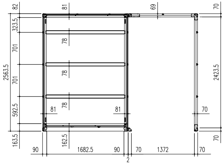
床伏図 (S = 1/50)
