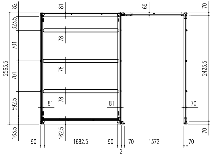
床伏図 (S = 1/50)
