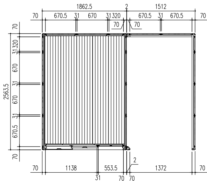
平面図 (S = 1/50)
