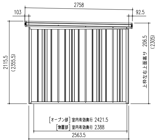
側面立面図 (S = 1/50) ※ ( ) 内寸法は、Hタイプを示す。
