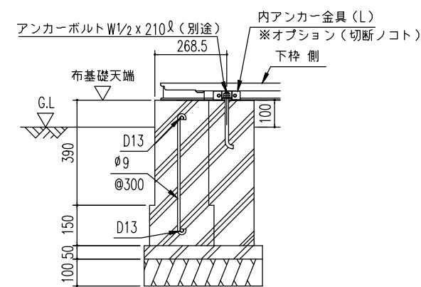
F ~ F' 断面
