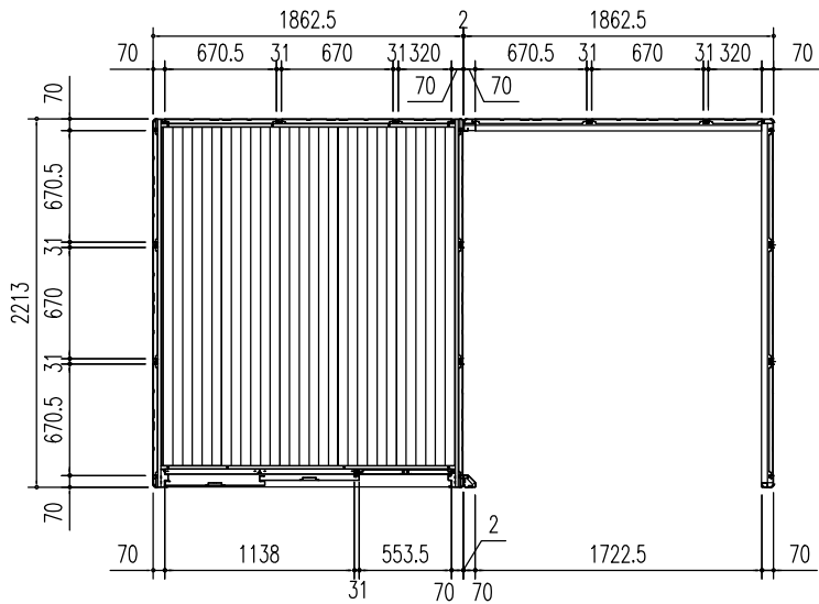
平面図 (S=1/50)
