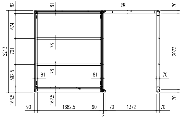
床伏図 (S = 1/50)
