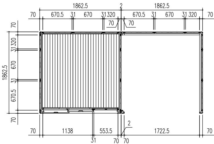
平面図 (S = 1/50)
