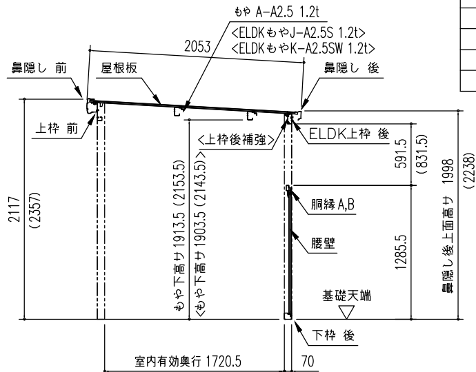
〔オープン部〕矩計図 (S = 1/50) ※ ( ) 内寸法は、Hタイプを示す。 ※ <>内は積雪型を示す。
