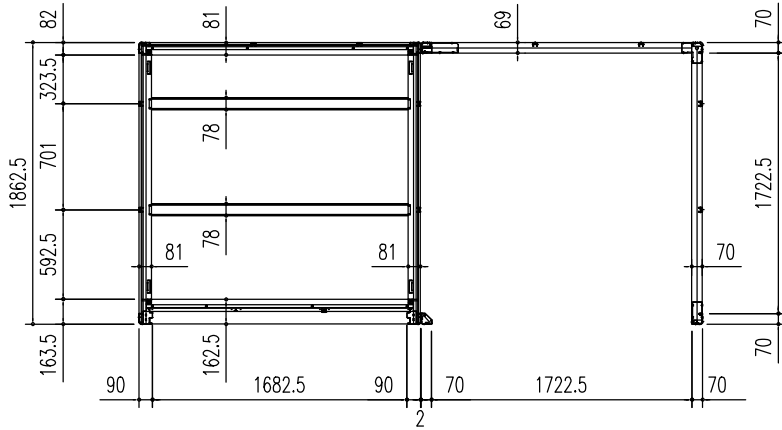
床 伏 図 (S = 1/50)
