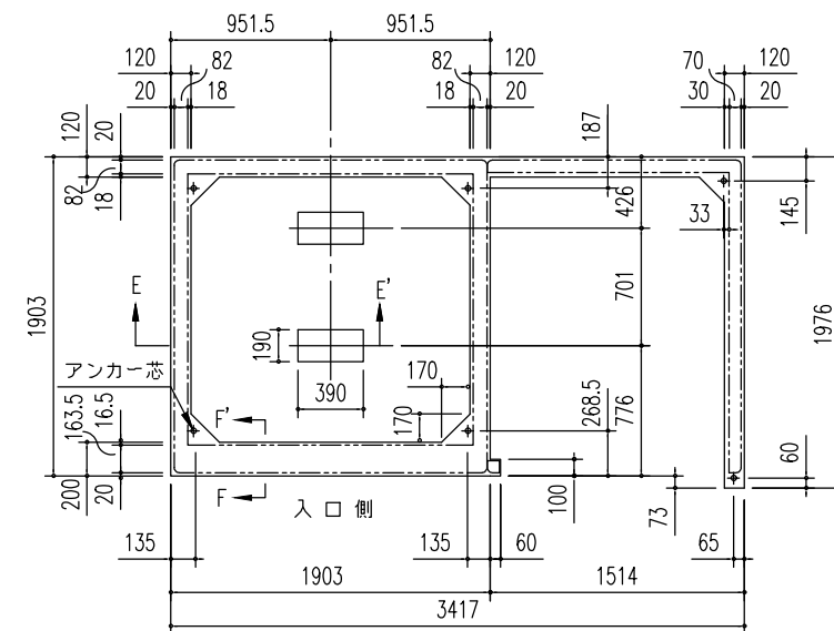
布基礎伏図 (S=1/50)
