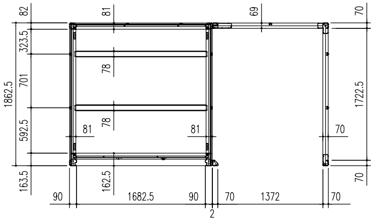
床伏図 (S = 1/50)
