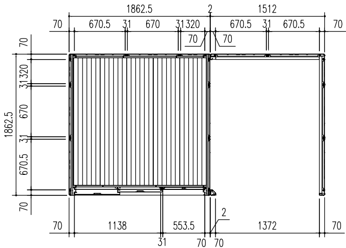
平面図 (S = 1/50)
