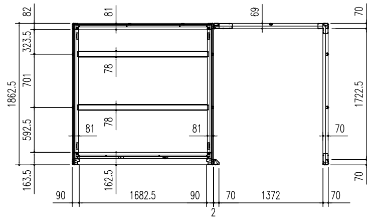
床伏図 (S = 1/50)
