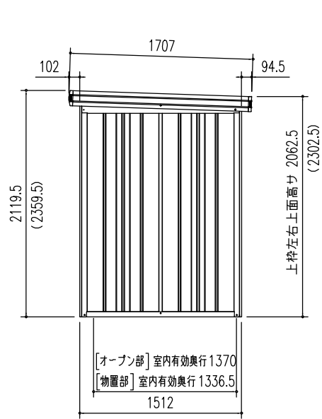
側面立面図 (S=1/50) ※ ( ) 内寸法は、Hタイプを示す。
