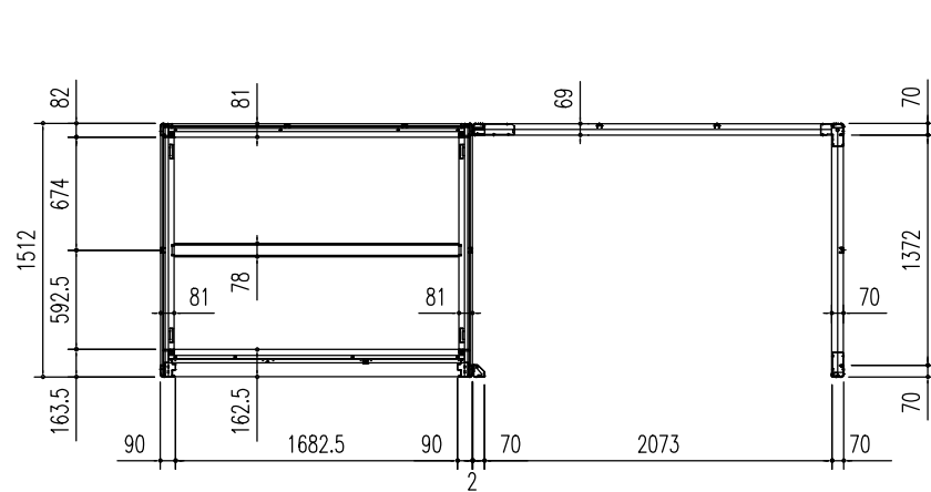
床伏図 (S=1/50)
