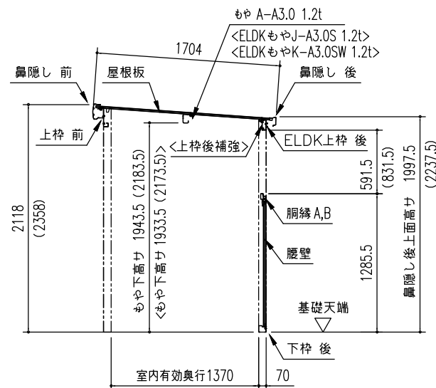
〔オープン部〕矩計図 (S=1/50) ※ ( ) 内寸法は、Hタイプを示す。 ※ <>内は積雪型を示す。
