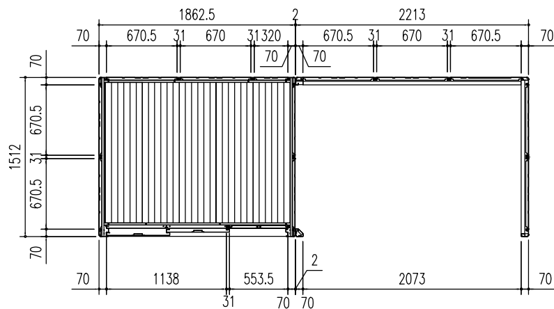
平面図 (S=1/50)
