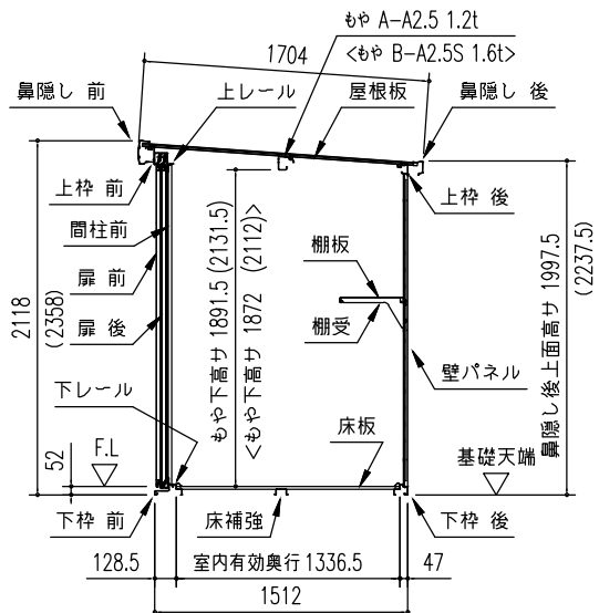
〔物置部〕矩計図 (S = 1/50) ※ ( ) 内寸法は、Hタイプを示す。 ※ <>内は積雪型を示す。
