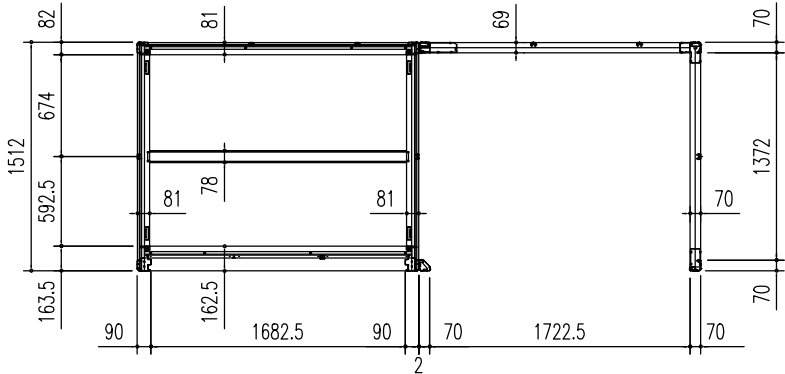
床伏図 (S = 1/50)
