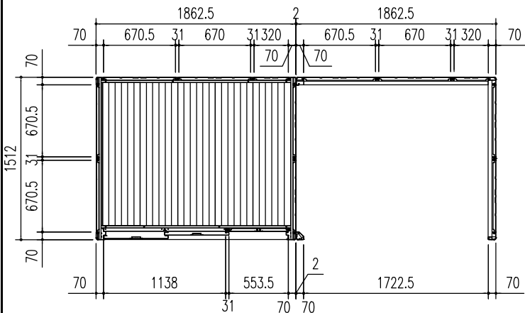
平面図 (S = 1/50)
