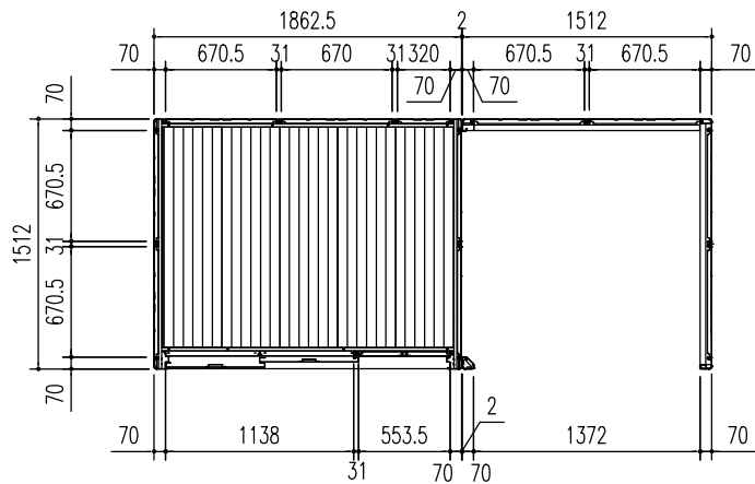
平面図 (S = 1/50)
