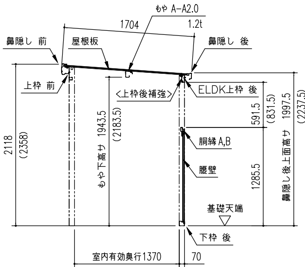
〔オープン部〕矩計図 (S = 1/50) ※ ( ) 内寸法は、Hタイプを示す。 ※ <>内は積雪型を示す。
