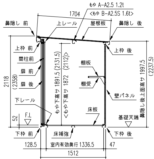
〔物置部〕矩計図 (S = 1/50) ※ ( ) 内寸法は、Hタイプを示す。 ※ <>内は積雪型を示す。
