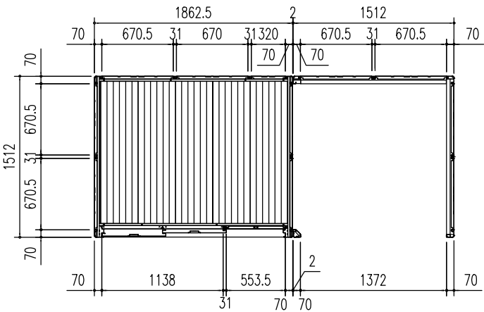
平面図 (S = 1/50)
