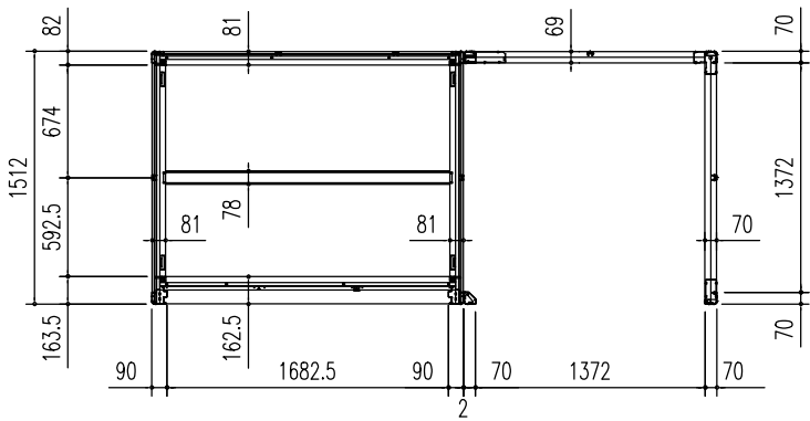
床伏図 (S = 1/50)
