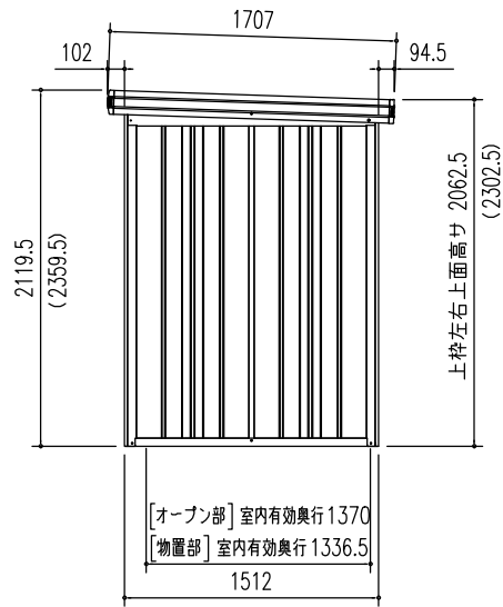
側面立面図 (S = 1/50) ※ ( ) 内寸法は、Hタイプを示す。
