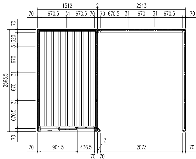
平面図 (S=1/50)
