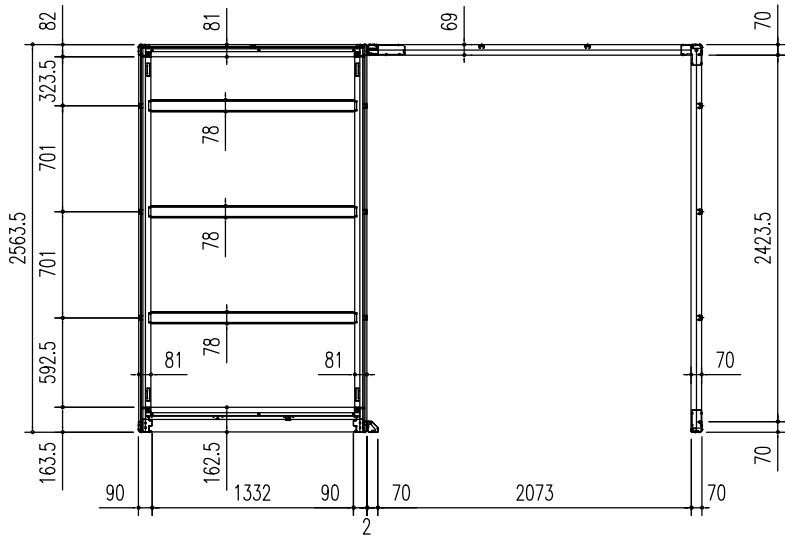
床伏図 (S=1/50)
