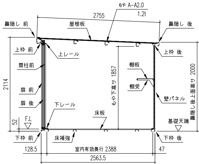
〔物置部〕矩計図 (S=1/50)
