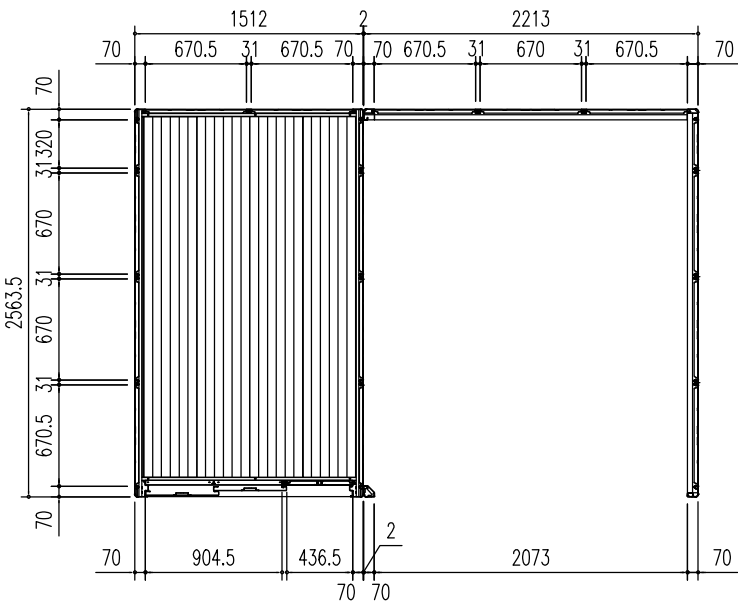
平面図 (S=1/50)
