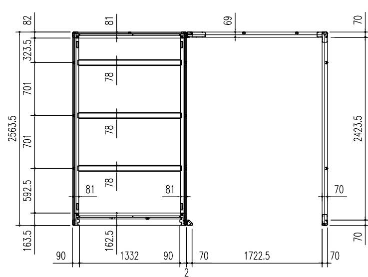
床伏図 (S = 1/50)
