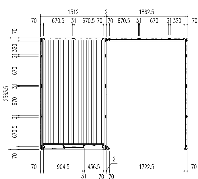
平面図 (S = 1/50)
