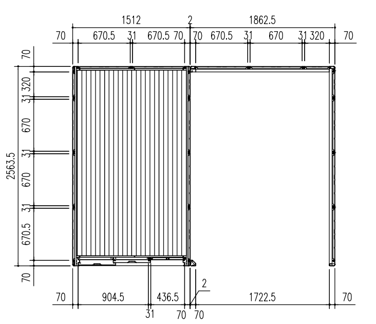
平面図 (S = 1/50)
