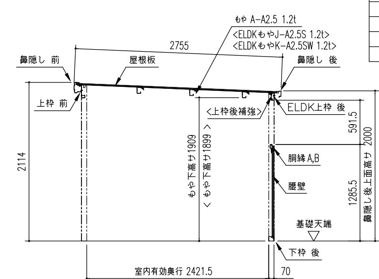
〔オープン部〕 矩計図 (S = 1/50)
