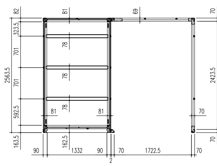
床伏図 (S = 1/50)
