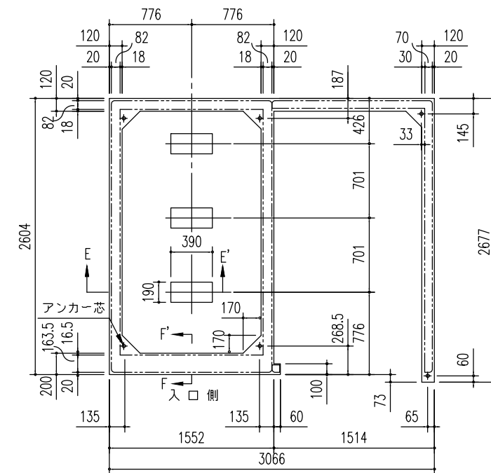
布基礎伏図 (S=1/50)
