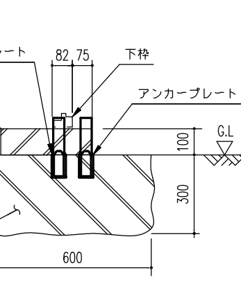
D ~ D' 断面 (外アンカー用)
