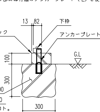
B ~ B' 断面 (外アンカー用)
