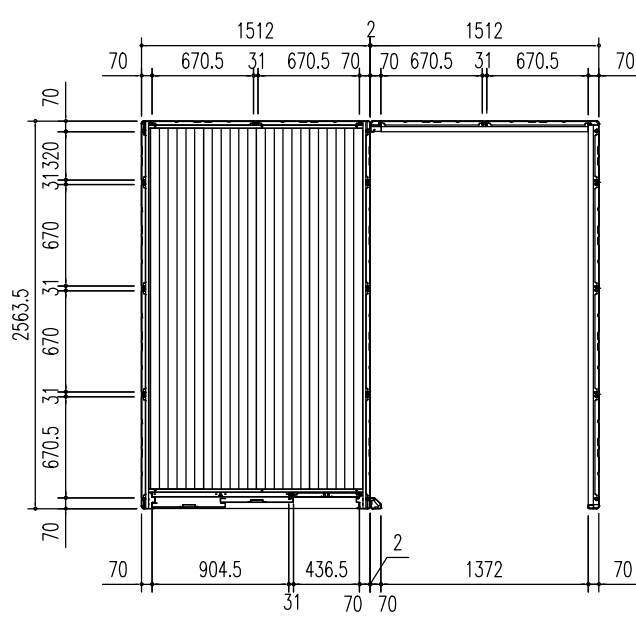
平面図 (S = 1/50)
