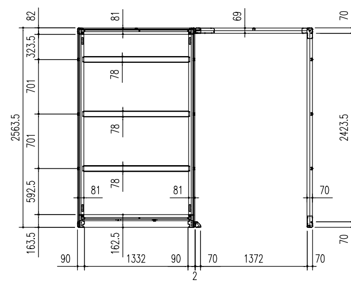
床伏図 (S = 1/50)
