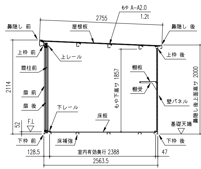
〔物置部〕矩計図 (S = 1/50)
