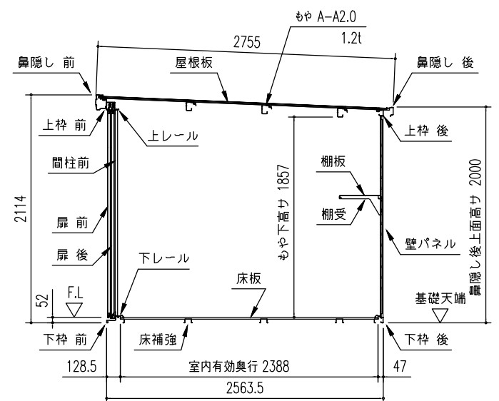
〔物置部〕矩計図 (S = 1/50) ※<>内は積雪型を示す。
