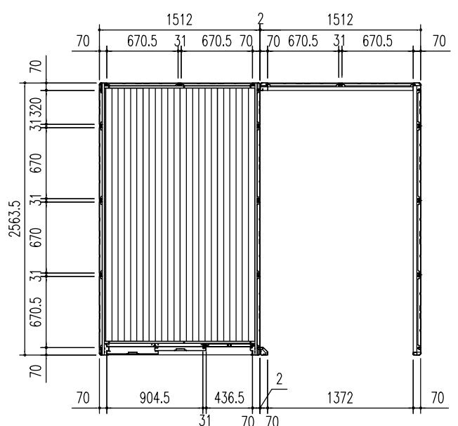
平面図 (S = 1/50)
