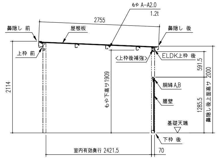
〔オープン部〕矩計図 (S = 1/50) ※<>内は積雪型を示す。
