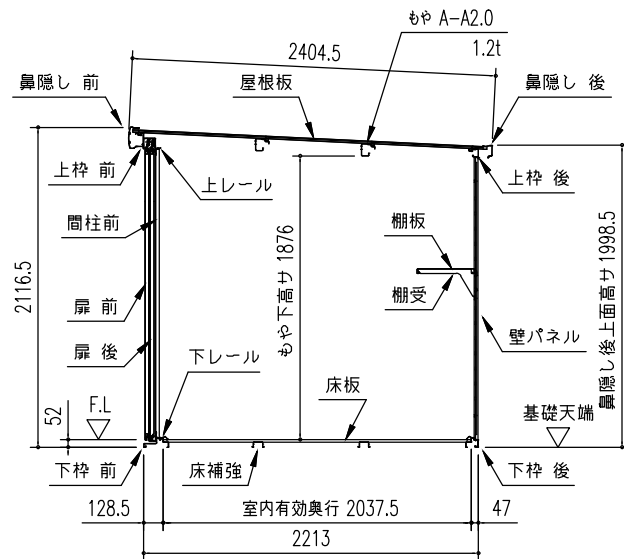
〔物置部〕 矩計図 (s = 1/50)
