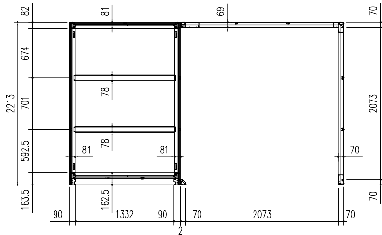
床伏図 (s = 1/50)
