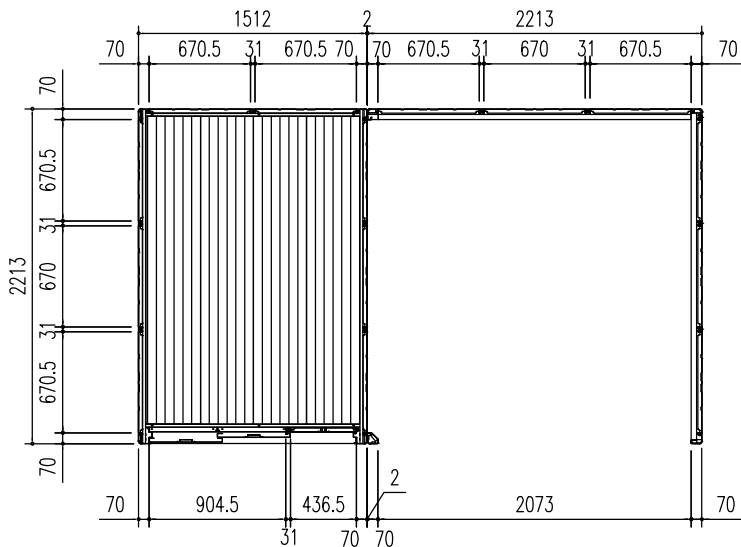
平面図 (s = 1/50)
