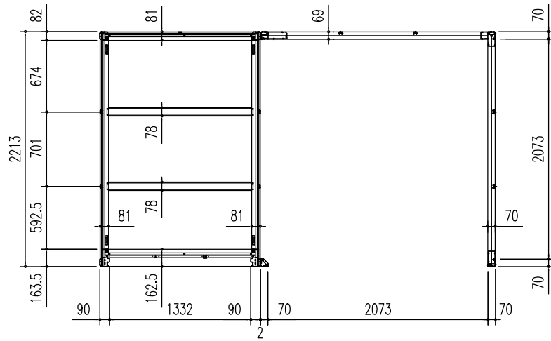
床伏図 (s = 1/50)
