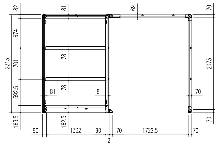
床伏図 (S = 1/50)
