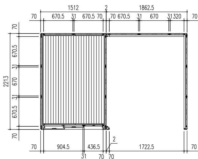
平面図 (S = 1/50)
