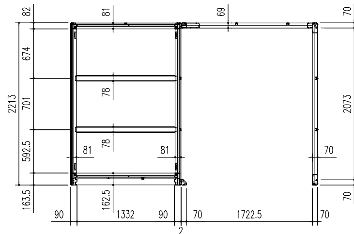
床伏図 (S = 1/50)
