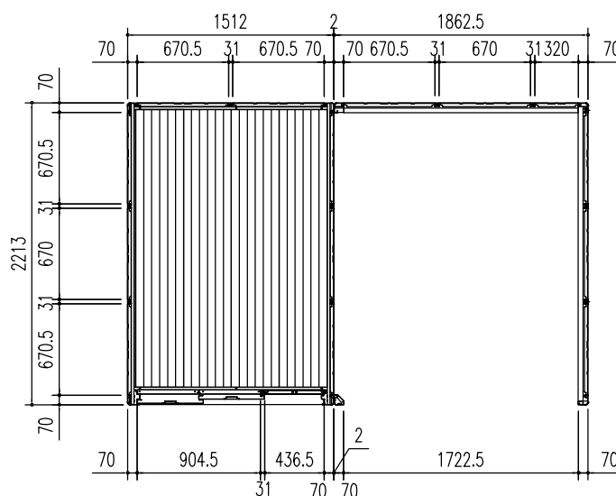
平面図 (S = 1/50)
