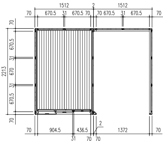
平面図 (S = 1/50)
