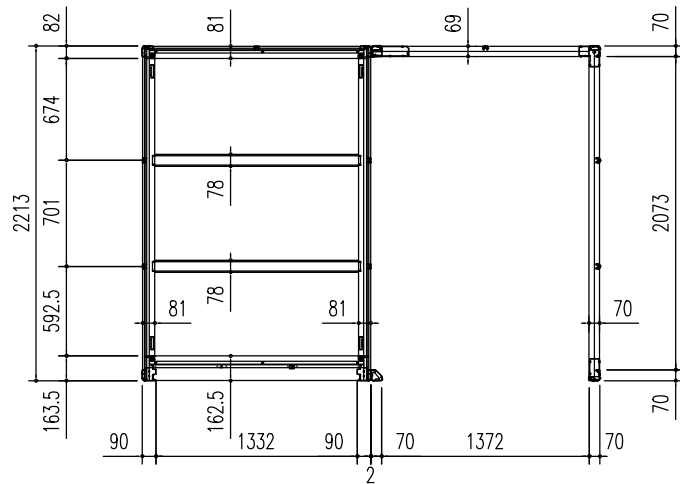
床伏図 (S = 1/50)
