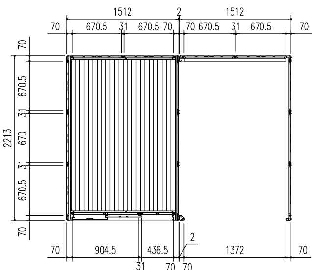
平面図 (S = 1/50)
