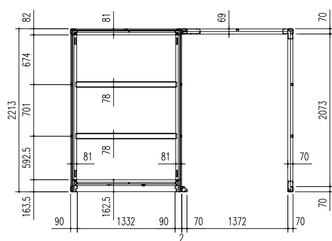
床伏図 (S = 1/50)
