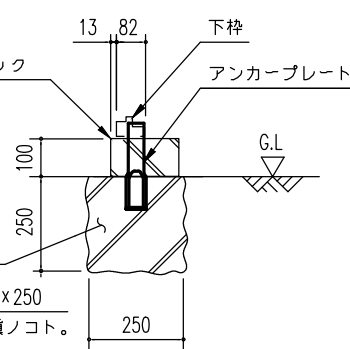
B ~ B' 断面 (外アンカー用)
