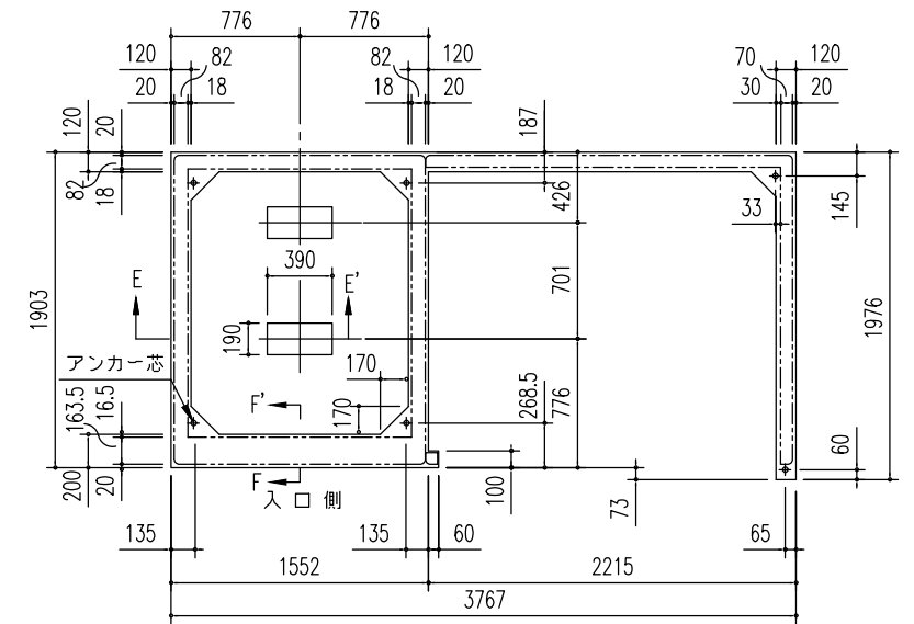
布基礎伏図 (S=1/50)
