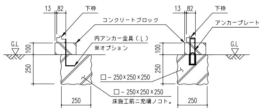
A ~ A' 断面 (内アンカー用)
