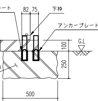
D ~ D' 断面 (外アンカー用)
